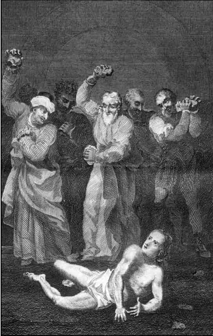
Stefanın daşlanması
